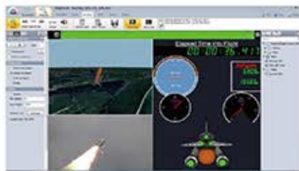
软件界面
